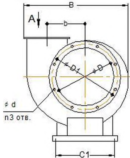
Схема расположения отверстий под фундаментные болты
