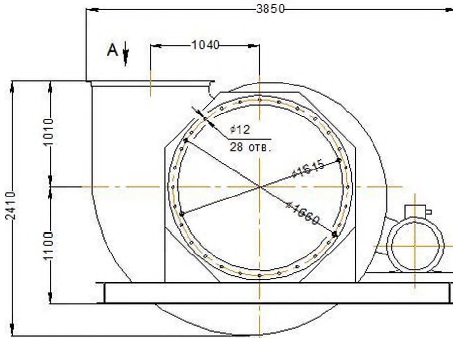
Положения корпуса вентилятора правого вращения
