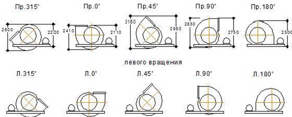
Положения корпуса вентилятора правого вращения
