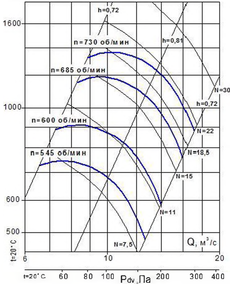
P_v , Па ВР 80-70-12,5 (исп. 1 и 5)
