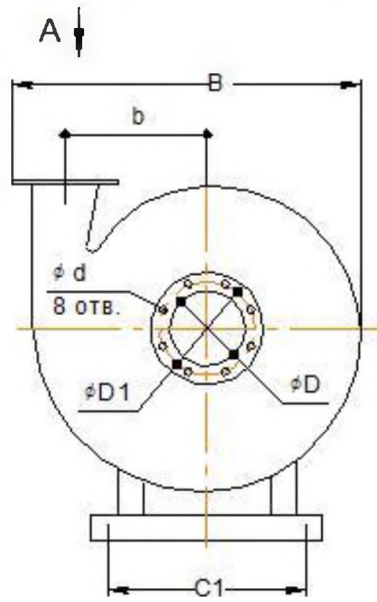
Схема расположения отверстий под фундаментные болты
